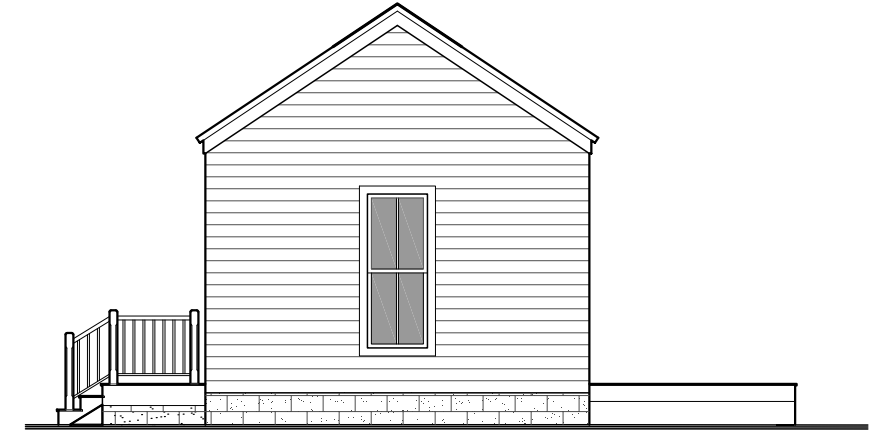
Right Elevation
