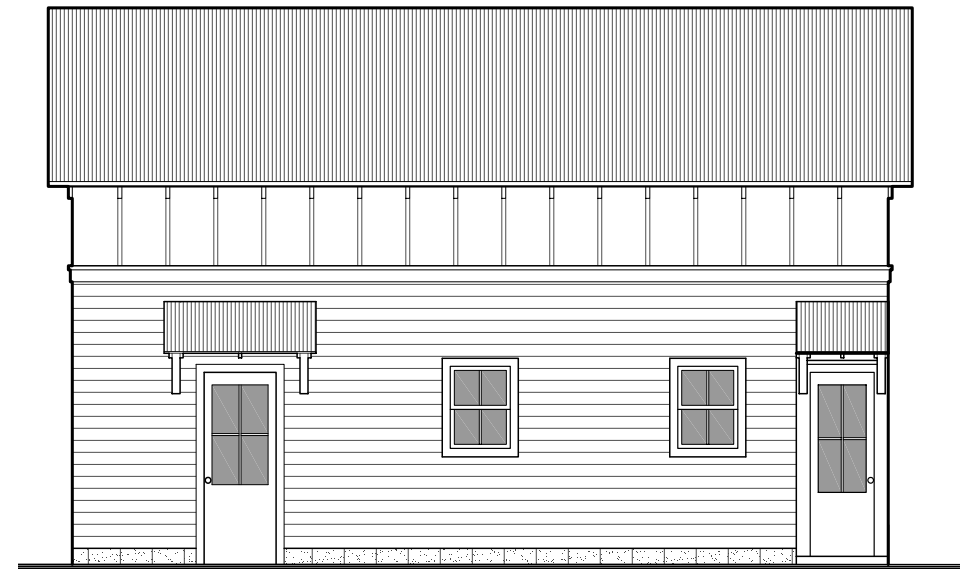
Right Elevation
